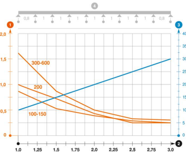
Diagramme de charge du chemin de câbles en treillis GRM 105
