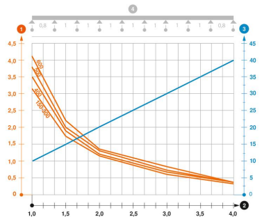
Diagramme de charge du chemin de câbles en treillis SGR 105
